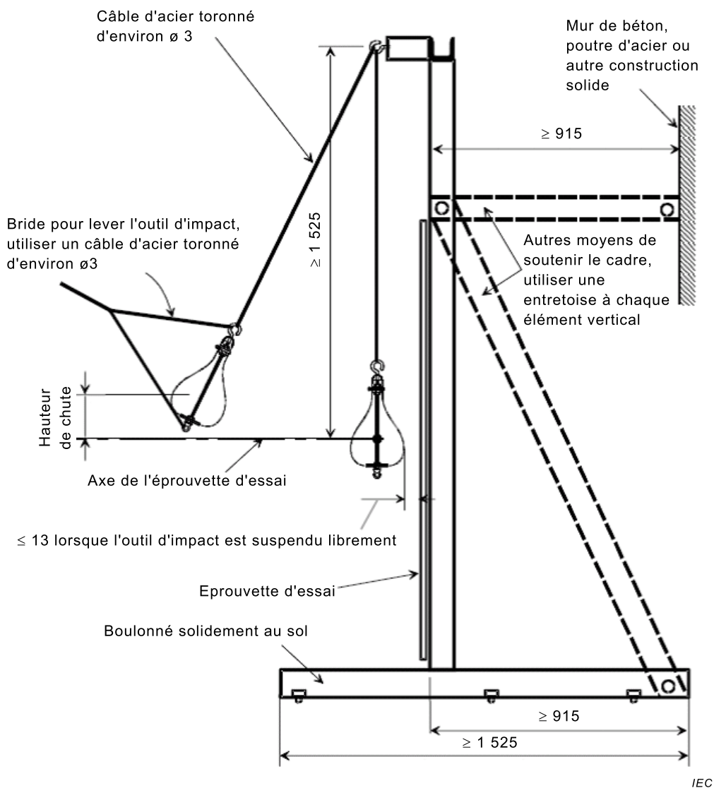
Figure 6 – Cadre d'essai d'impact 1
